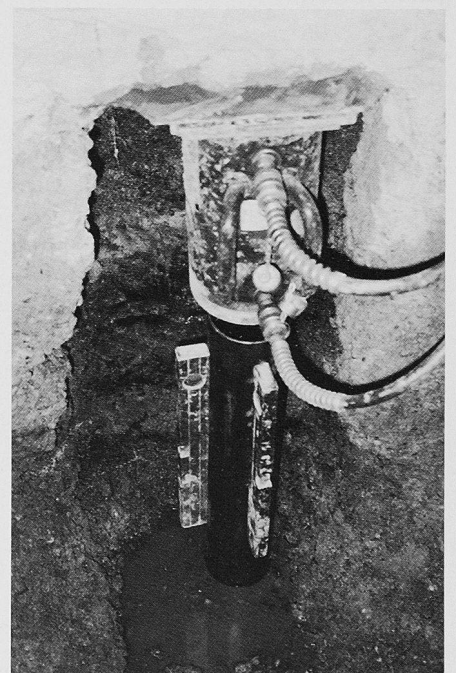
Bild 7. Presspfähle, Objekt Birmensdorferstr. 326, Zürich (alle Bilder: Tertratech AG)
