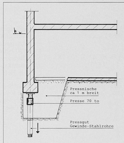
Bild 2. Presspfahl
