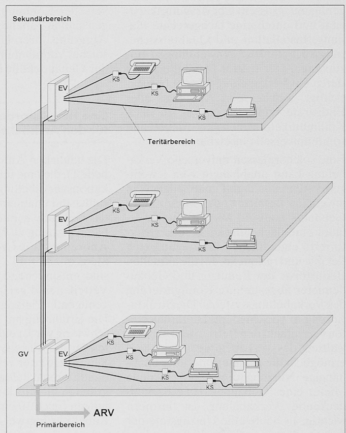
Bild 2. Hierarchische Sternstruktur einer universellen Kommunikationsverkabelung: Arealverteiler (ARV), Primärsektor, Gebäudeverteiler (GV), Sekundärsektor, Etagenverteiler (EV), Tertiärsektor, Kommunikationssteckdose (KS)
