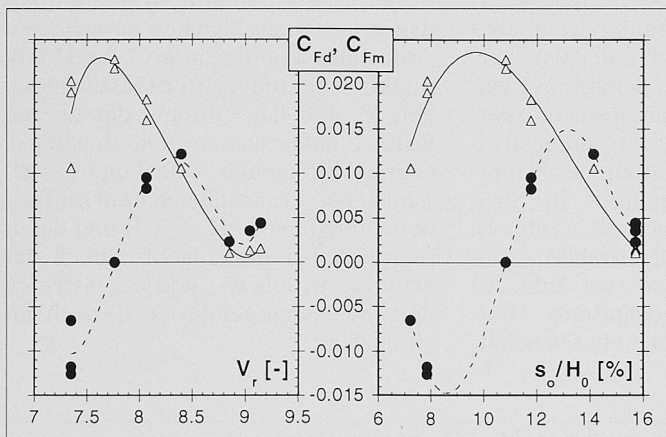
Bild 9. Anfachungskoeffizienten (●) C_{Fm} und (Δ) C_{Fd} für die vertikale Starrkörperbewegung z(t) : a) in Funktion der reduzierten Geschwindigkeit V_r , b) in Funktion der relativen Öffnung der oberen Schütze s_o/H_0
