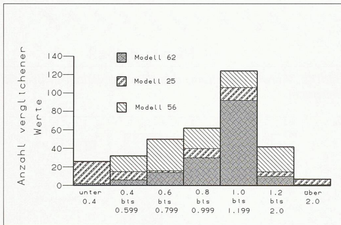
Bild 9. Verschiebung [TH mit U]/Verschiebung [RS mit U]. Modelle in Basislage
