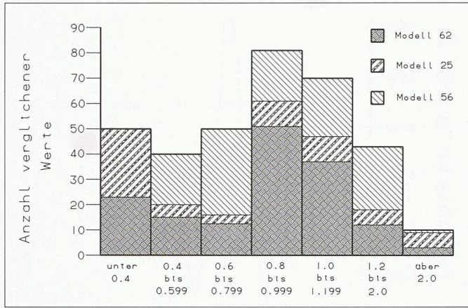
Bild 7. Verschiebung [TH mit MSE]/Verschiebung [RS mit MSE]. Modelle in Basislage
