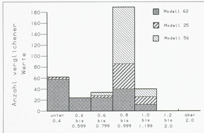
Bild 5. Verschiebung [TH mit MSE]/Verschiebung [TH mit U]. Modelle in Basislage
