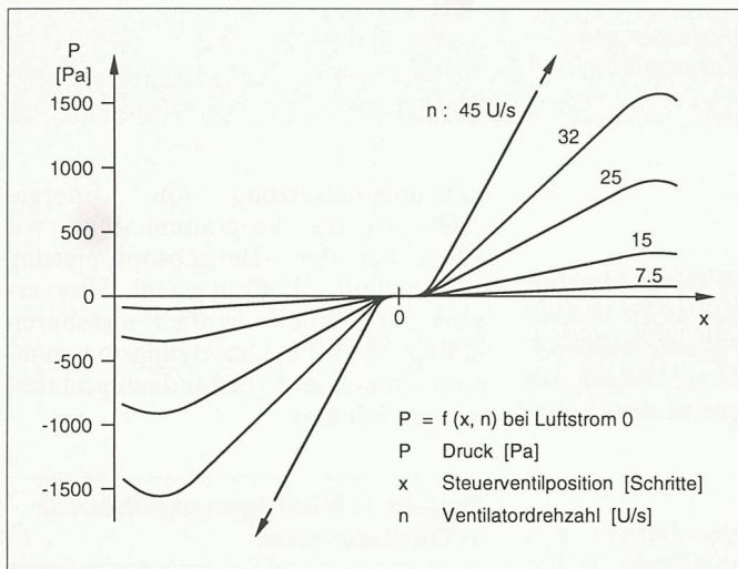
Bild 2. Steuerventilcharakteristiken (SVC)
