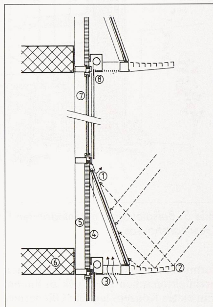
Bild 1. Schnitt durch Fassadenkonstruktion eines Bürogeschosses. 1 – Photovoltaik; 2 – Reflektierende Chromstahl-lamellen; 3 – Hinterlüftung; 4 – Thermische Isolation; 5 – Pfosten-Riegel-Metallkonstruktion; 6 – Geschossdecke; 7 – Metallfenster; 8 – Stoffrollo
