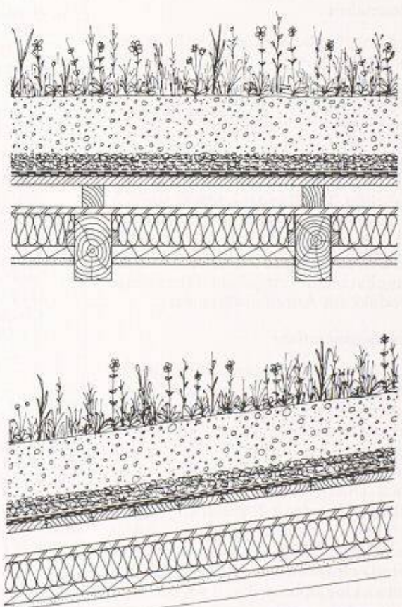
Bild 4. Umkehrdach, Beispiel des Gründachaufbaues in 2 Varianten
