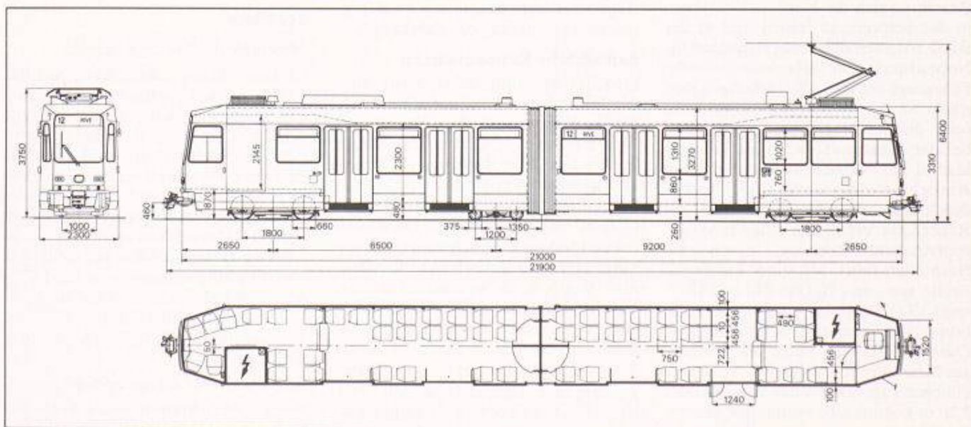
Bild 4. Niederflurtram der Genfer Verkehrsbetriebe (Typ 2), Zeichnung ACMV Vevey.
