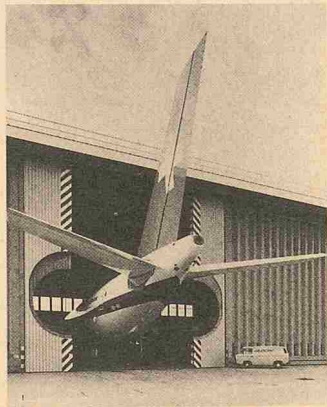
Gilgen-Hangartorantrieb
