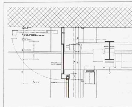
Detailschnitt
