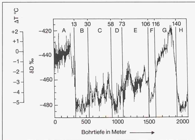
Bild 14. Jouzel et al. [3] untersuchten das Alter eines Eisbohrkerns von Vostok (Antarktis) anhand der Deuteriumkonzentration. Das Defizit an Deuterium \delta D wird in Promillen angegeben. Ganz links zeigt eine ungefähre Skala, wie stark die Temperaturen in der gemässigten Zone der nördlichen Halbkugel durchschnittlich sanken. Die horizontale Skala gibt an, aus welcher Tiefe die analysierte Bohrprobe stammt, die Ziffern oben geben das Alter in tausend Jahren an.
