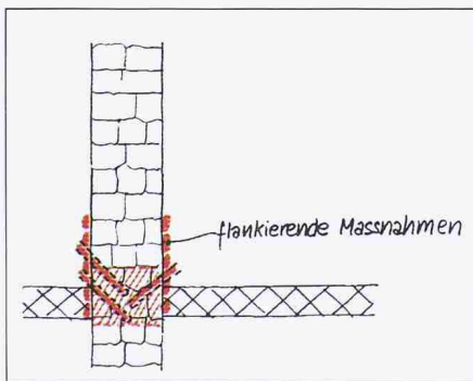
Bild 4. Horizontalsperre für Zwischenwände
