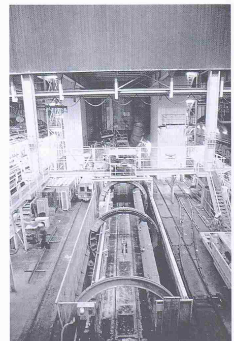
Bild 10. Entlad der mit Tunnelausbruch beladenen Züge mittels Rotationskipper im Sangatte-Schacht (Photo Ph. Demail)
