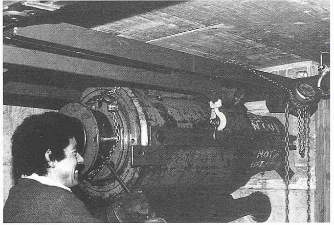
Bild 9. Spannpressen mit Hebevorrückung
