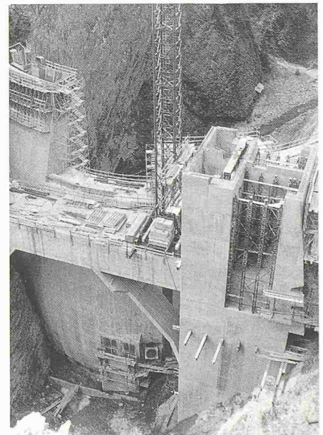
Naturgemäss kann die Schweiz als Bergland ihre Wasserkraft gut nutzen. Mit einem Anteil von über 60% liegt sie weit über dem EG-Durchschnitt. Im Bild der Bau der Staumauer Solis im Bündnerland, wo seit einigen Jahren die Wasser der Albula gestaut werden (Bild: Comet)
