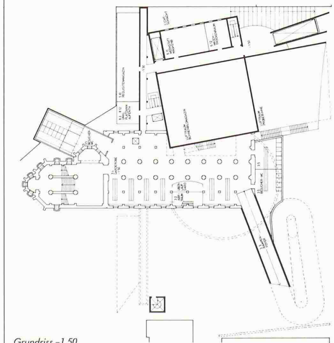
Grundriss -1.50
