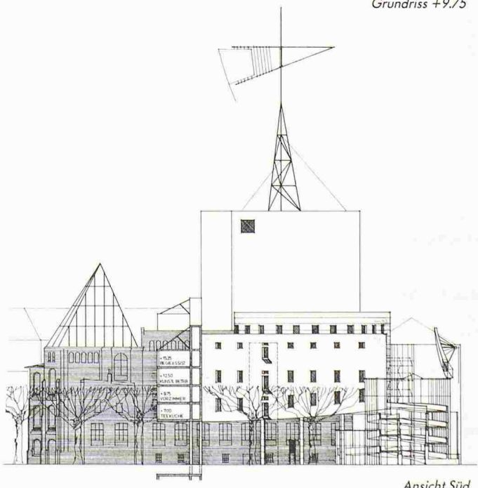
Ansicht Süd
