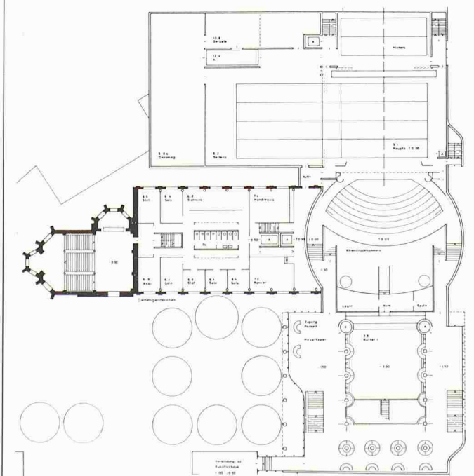
Parkett/Bühnengeschoß
