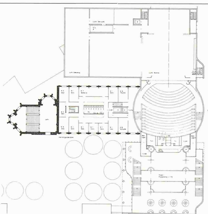
Parkett-, Bühnengeschoß
