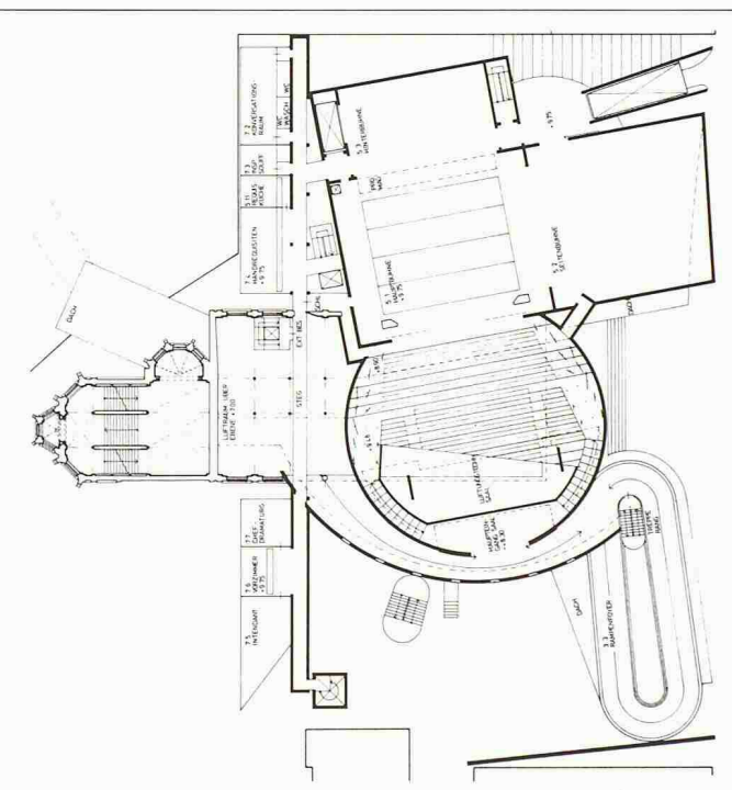
Grundriss +9.75
