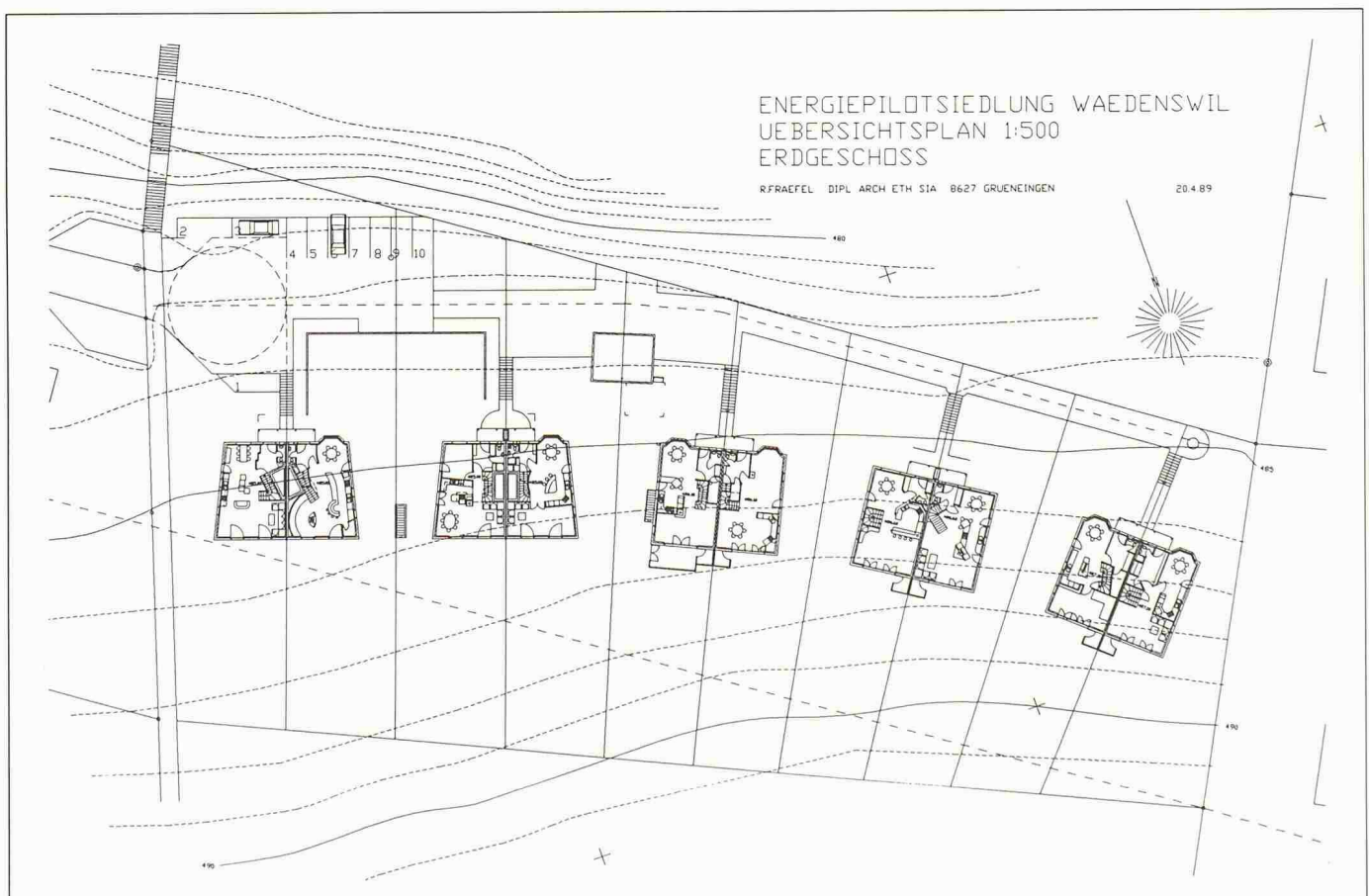
Bild 1. Anordnung der 10 Doppel Einfamilienhäuser auf dem in Ost-West-Richtung langgezogenen Grundstück
