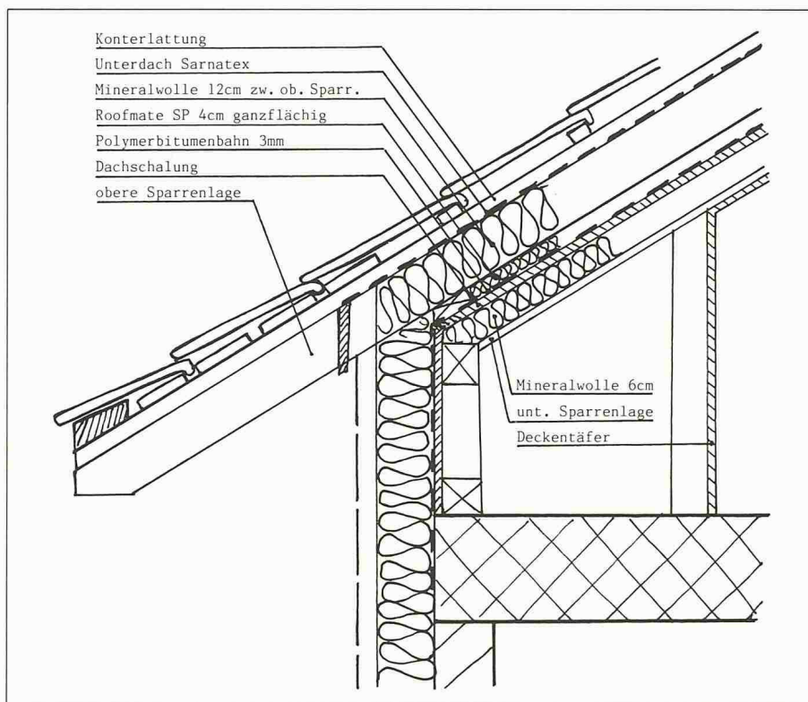
Bild 2. Konstruktion des luftdichten Dachaufbaus
