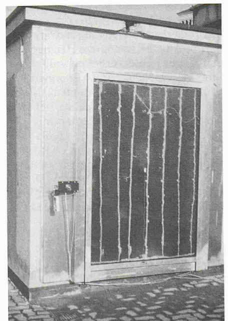
Bild 4. Testkollektor von 2,5\text{ m}^2 Fläche, am Liftaufbau des Amts für technische Anlagen und Lüfthygiene montiert.
