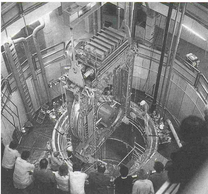
Eine supraleitende Magnetspule mit einer für künftige Fusionsreaktoren typischen Grösse wird in den Kryostaten eingefahren, in dem sie bei einer Temperatur von -269^{\circ}\text{C} betrieben wird
