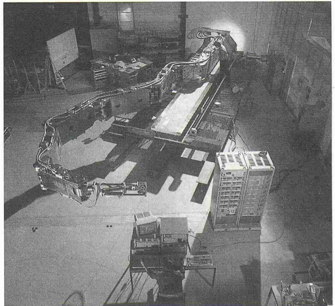
Für den Einsatz bei Wartungsarbeiten im Tokamak-Testreaktor in Princeton, USA, wurde dieser 9 Meter lange rechnergesteuerte Manipulatorarm entwickelt (Bild: KfK)
