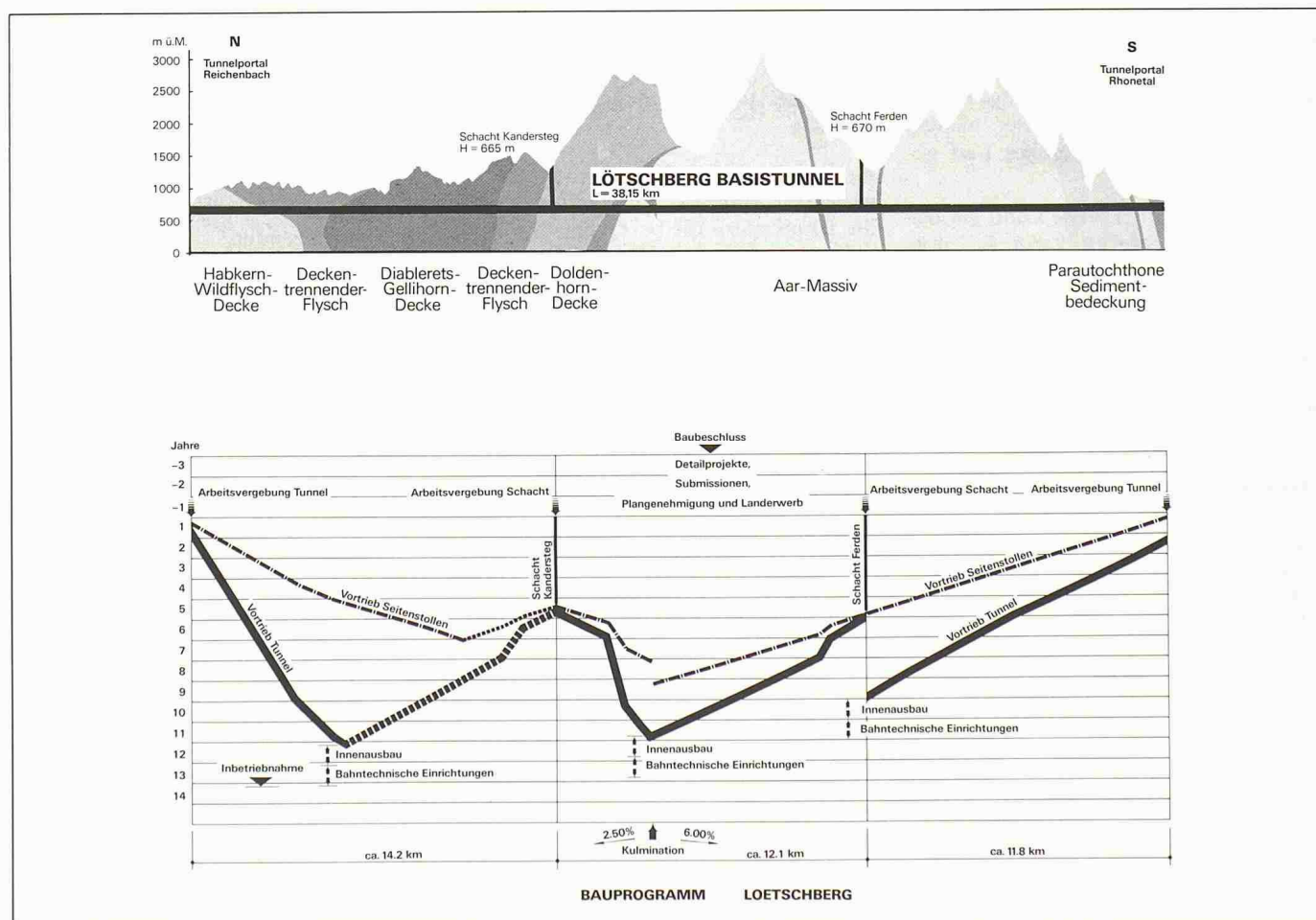
Bild 4. Bauprogramm Lötschberg-Basistunnel
