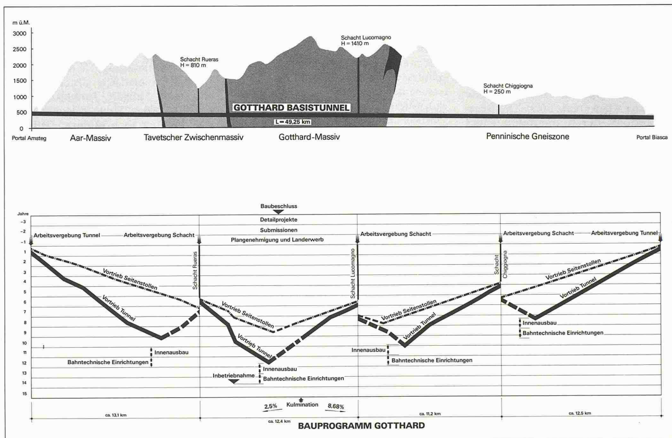
Bild 3. Bauprogramm Gotthard-Basistunnel
