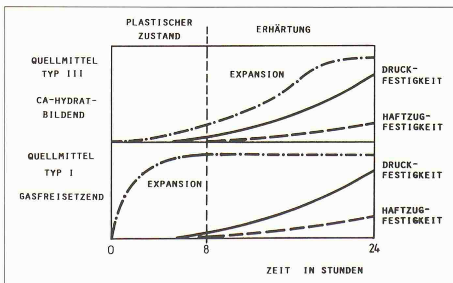
Bild 4. Vergleich des Expansionsverhaltens von Beton mit einem gasfreisetzendem Quellszement (Typ I) und einem langsam wirkenden Expansionsmittel (Typ III). Das gasfreisetzende Material (unten) wirkt nur während weniger Stunden bis zum Abbindebeginn des Betons. Ein Spannungsaufbau ist nicht möglich. Das langsam wirkende Mittel (oben) auf der Basis von \text{CaO} hydratisiert während der Festigkeitsentwicklung. Da der Beton bereits an der Armierung haftet, können Druckspannungen im Beton aufgebaut werden
