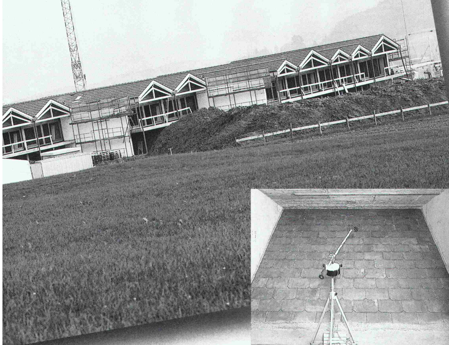
Luftschallprüfung am Grossmodell EMPA Zürich
