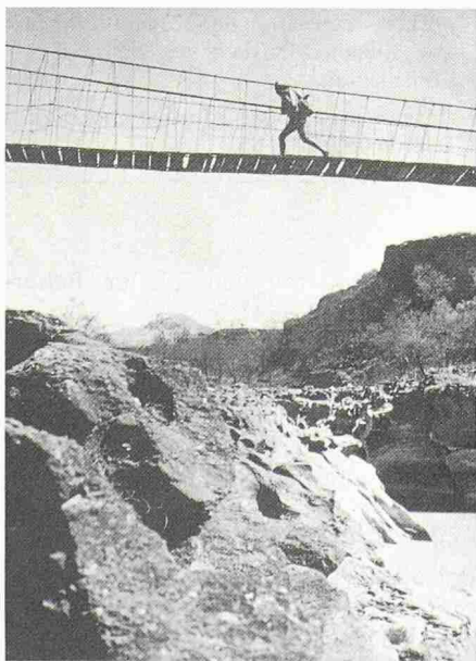
Bild 3. Hängebrücke bei Hilitar, Westnepal. Im Rahmen der nepalesisch/schweizerischen Entwicklungszusammenarbeit sind in den letzten 25 Jahren über 200 grössere Fussgängerbrücken mit Spannweiten bis zu 300 Metern gebaut worden. (DEH-Fotothek/Max Lehmann)
