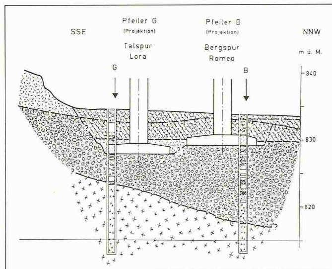
Bild 6. Geologisches Querprofil G-B
