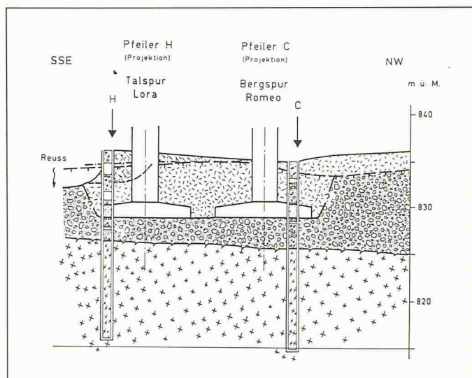
Bild 5. Geologisches Querprofil H-C
