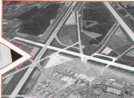
Betonimprägnierung
