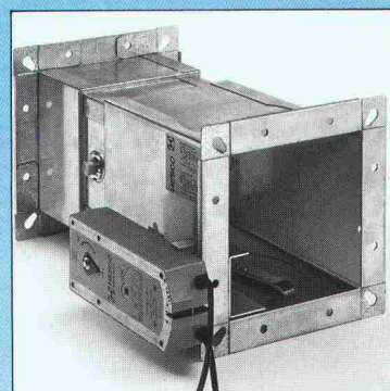
Brandschutzklappen
