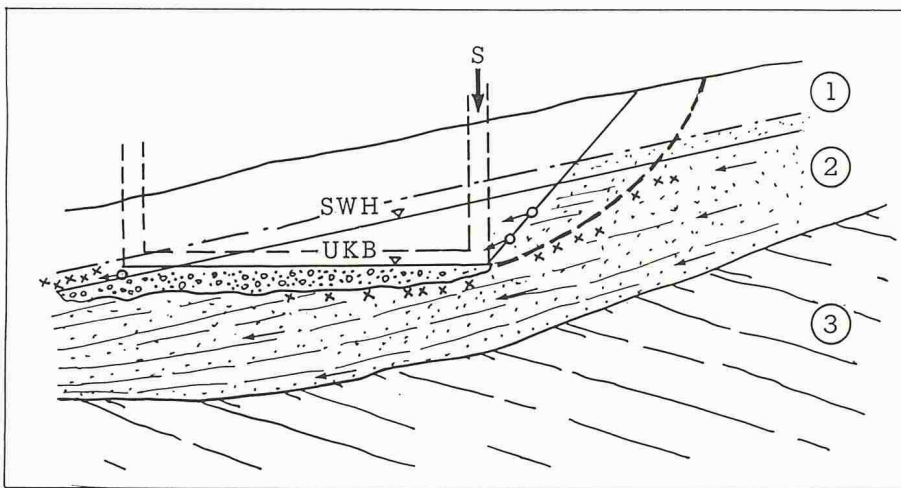
Bild 6. Gegenüberstellung eines Bauvorhabens mit gegebener Sickerwassersituation. SWH = Sickerwasserhorizont, UKB = Unterkannte Bauwerk, 1 = Verwitterte Deckschicht, 2 = Randeiszeitliches Schwemmsediment, 3 = Molasse-Sandstein, x x x = Feinstofftransport
