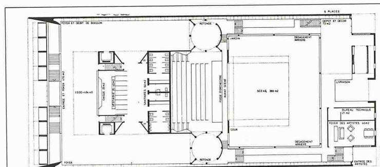
Rez-de-chaussée 1:750
