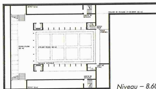
Niveau - 8.60
