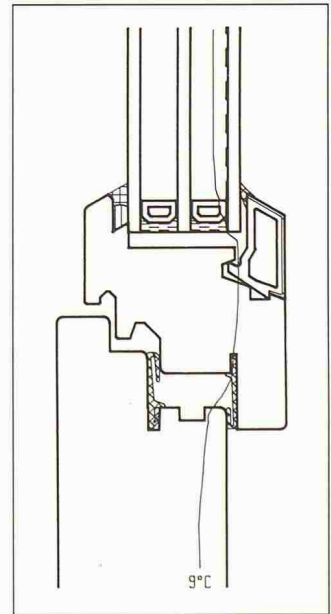
Bild 10. Detail B4, entspricht Detail B3, jedoch ist die Kunststoff-Glashalteleiste auf ihrer sichtbaren Fläche mit einem wärmeleitenden Überzug aus Aluminium und einem wärmeleitenderen Dichtungsprofil versehen
