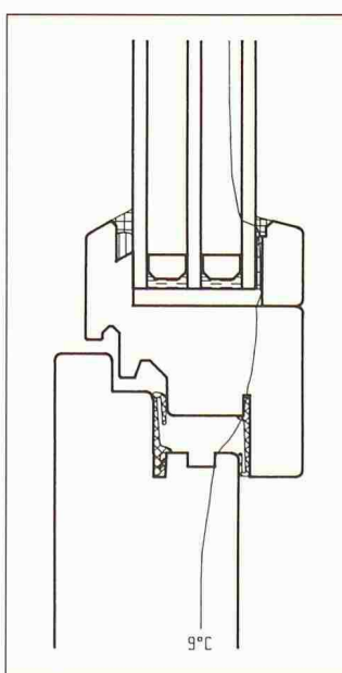
Bild 5. Detail A3, das heisst mit Vergrößerung der Glasfalzhöhe von 18 auf 25 mm
