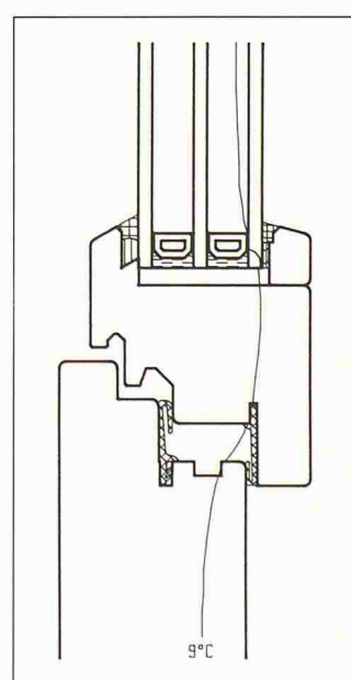
Bild 6. Detail A4, entspricht in Konstruktion dem Detail A2, jedoch Isolierglas-Randverbund mit Distanzstegen in Kunststoff statt Stahl
