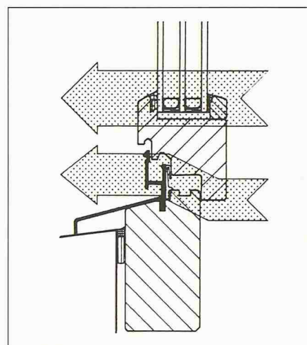
Bild 1. Wärmebrücken am Fenster
