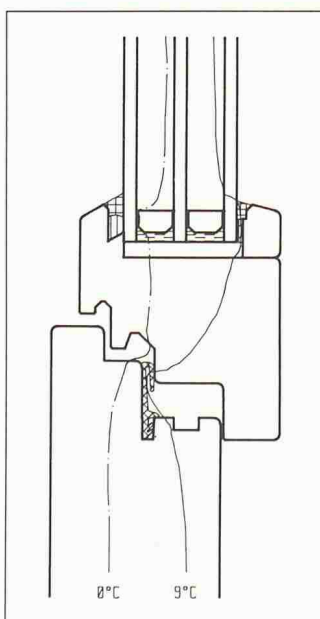
Bild 3. Konstruktion A1, Standard-Holzfenster mit Mitteldichtung
