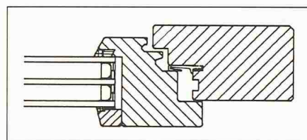
Bild 2. Schnittdetail seitlich
