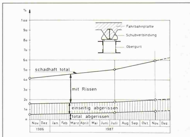
Bild 9. Entwicklung der Schweissnaht-Risse an den Schubverbindungen
