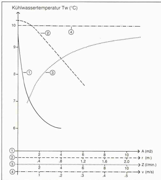
Bild 6. Innenluft- und Kühlwassertemperatur in Abhängigkeit von Geometrie, Wasserzufluss und Windgeschwindigkeit [Variable Parameter: 1: Wasseroberfläche A ( m^2 ). - 2: Innenradius r (m). - 3: Quellwasserzufluss Z (l/min.). - 4: Windgeschwindigkeit v (m/s). - Konstante Parameter: 2,3,4: A = 2 \cdot 2 \cdot \pi . - 1,3,4: r = 2 . - 1,2,4: Z = 1.5 . - 1,2,3: v = 0.1 ]
