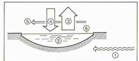
Bild 4. System Kühlwasser [1: Quellwassertemperatur TQ. - 2: Kühlwassertemperatur T_w . - 3: Verdampfungs-Kühlleistung K_w . - 4: Wärmeabgabe des Luftkörpers an das Kühlwasser. - 5: Luftgeschwindigkeit v. - 6: Wasseroberfläche A]
