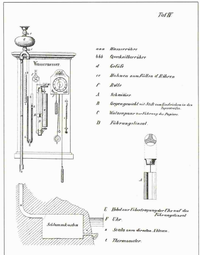
Bild 2. Limnigraf, «Differentialhebergerät» von A. Gressly, Solothurn [5]
