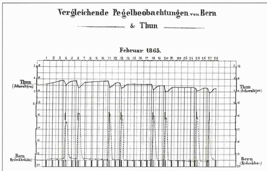
Bild 3. Schwallmessungen an der Aare zwischen Thun und Bern. Oben die Ganglinie (ausgezogen) des Pegelstands in Scherzligen am Auslauf des Thunersees; unten die Ganglinie (punktiert) des Pegelstands an der Nydeggbrücke in Bern. Pegelskala in Fuss, Pegelhorizonte ungleich. An zwei Fahrtagen pro Woche wurde mit den Thuner Staatsschleusen ein Schwall zur Erleichterung der Schifffahrt und Flösserei erzeugt [5]
