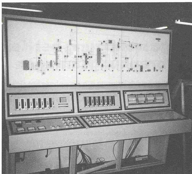
Bild 9. Schaltwarte der LUBREX TM -Anlage in Neuseeland
