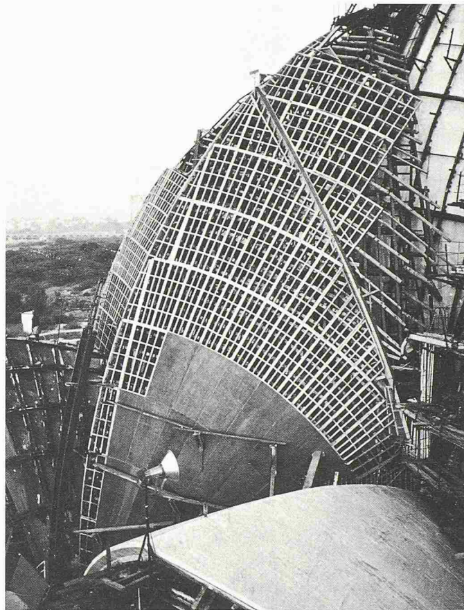
Bild 10. Schalung der «Äusseren Blätter»
