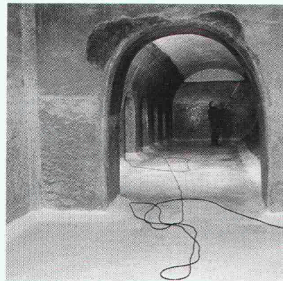
Wasserreservoir Muttenszwald: Kombination von verschiedenen Sanierungs-Methoden: Injektionen gegen eindringendes Wasser und zur Verfestigung des Gewölbes, Auskleidung durch starre Abdichtung.
