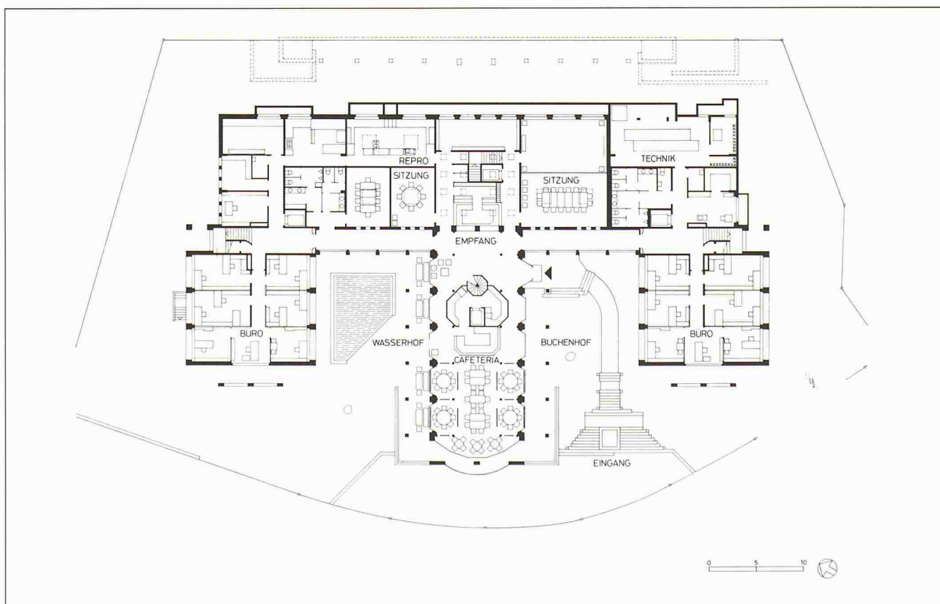
Bild 12. Grundriss Eingangsgeschoss
