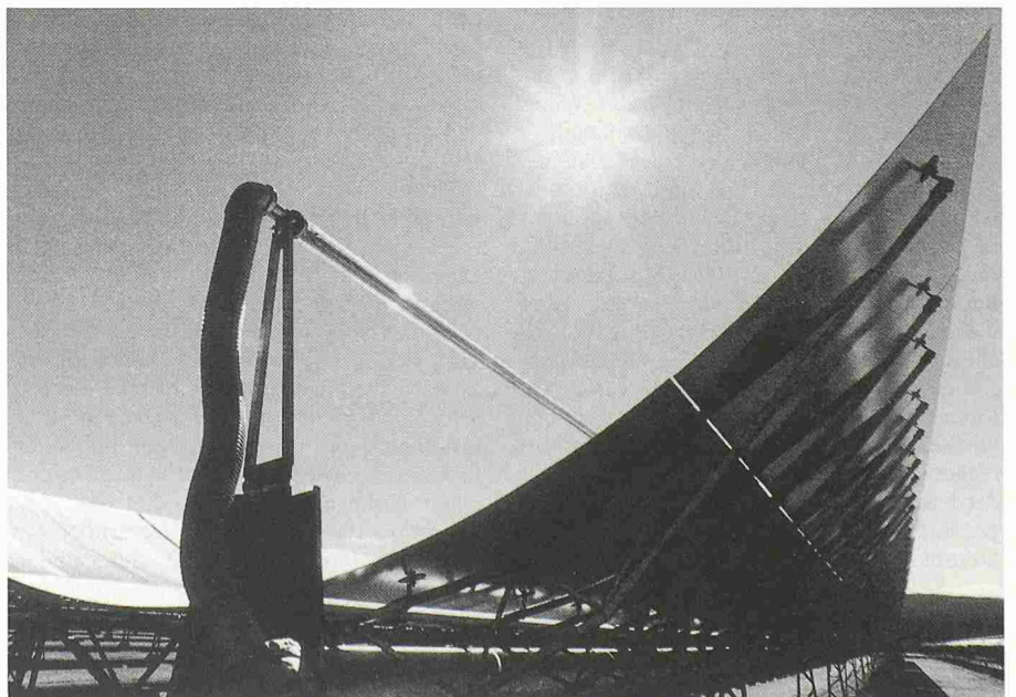
Aus der Schweiz kommen die zwei 35-MW-Dampfturbinengruppen für die beiden derzeit grössten Solarkraftwerke der Welt, die in der Nähe von Los Angeles gebaut werden (Bild: Asea Brown Boveri, Baden)
