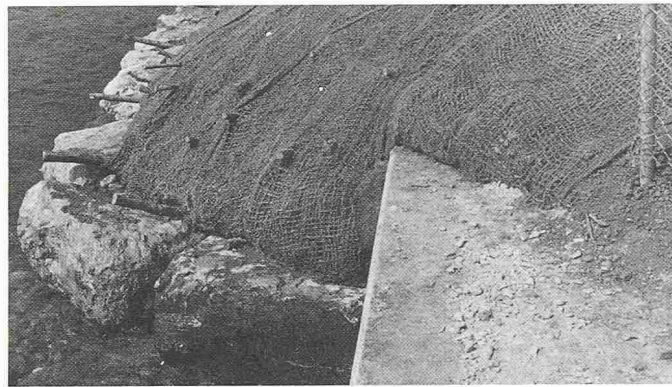
Bild 4. Detail mit Weidensteckhölzern und Juteabdeckung
