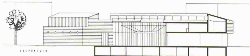
Schnitt Fussgängerpassage
