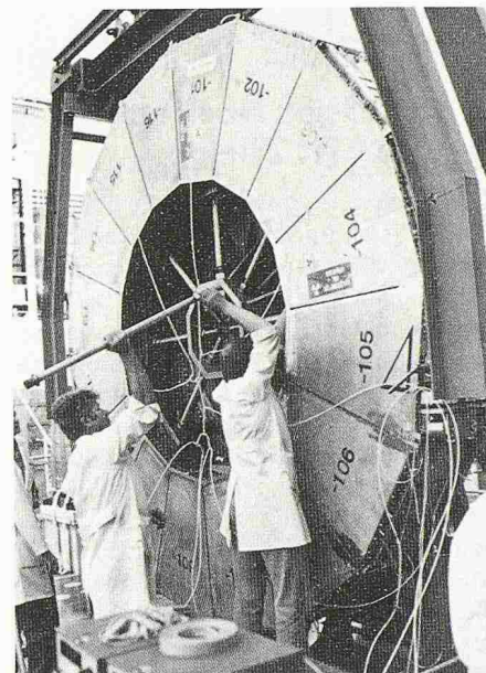
Bild 4. Hadron-Kalorimeter. 16 Module bilden einen Ring. Das Kalorimeter besteht aus 9 Ringen
