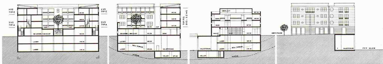
Querschnitt B-B
