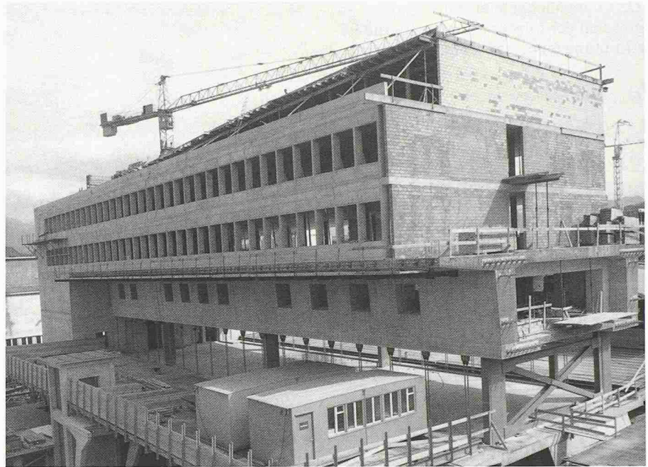
Bild 6. Gesamtübersicht mit Brücke im Bauzustand, ganz unten die aufgehängte Zwischendecke über EG (Foto E. Kneubühler, Kriens)
