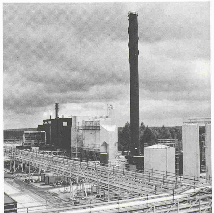
Bild 5. General Electric, Waterford/N.Y., USA: Die Anlage ist zur Verbrennung von festen, halbfesten und flüssigen Industrieabfällen geeignet. Die Leistung beträgt 1 \times 10 MW, und es ist keine Wärmeverwertung vorhanden. Inbetriebsetzung: 1980
