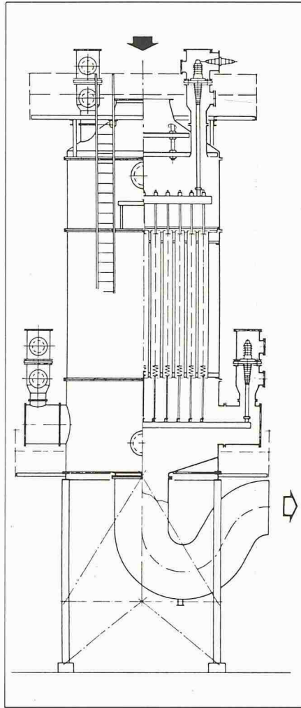
Bild 5. Nasselektrofilter
