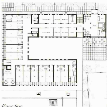
Piano tipo
