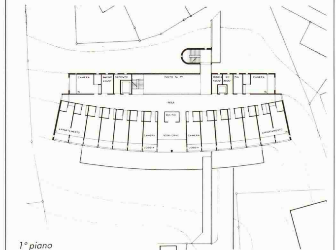
1° piano
