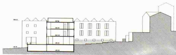
Sezione C
