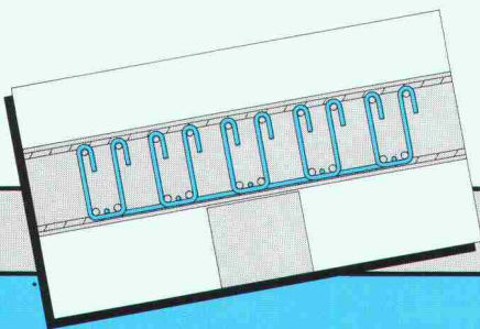
Anordnung der Bewehrung bei einem Dura-Durchstanzkorb
