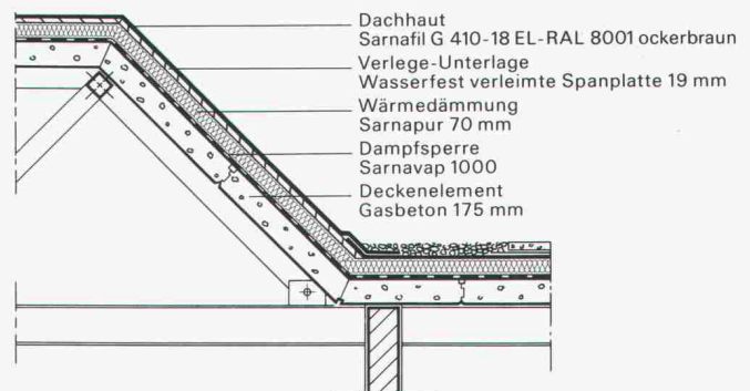
Übergang vom bekieseten Flachdach zum farbigem Sarnafil-Shed.
