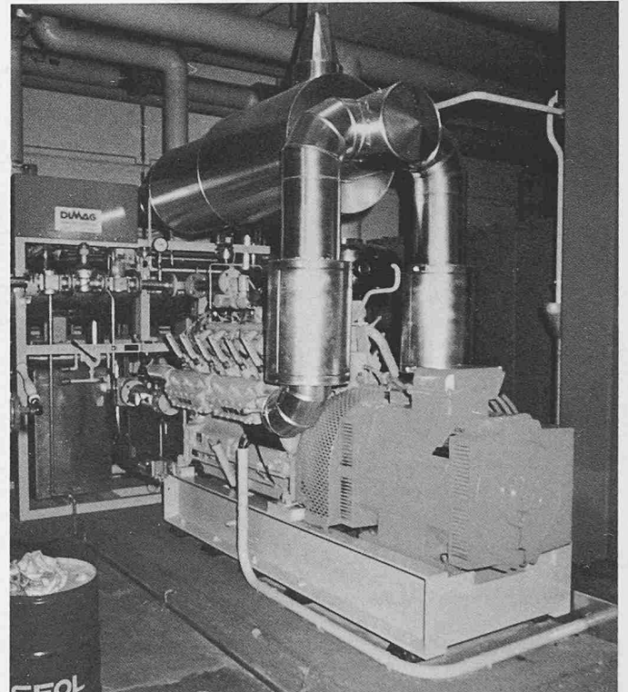
Bild 3 (rechts). Blockheizkraftwerk Überbauung Holeeholzacker, Binningen, BL
