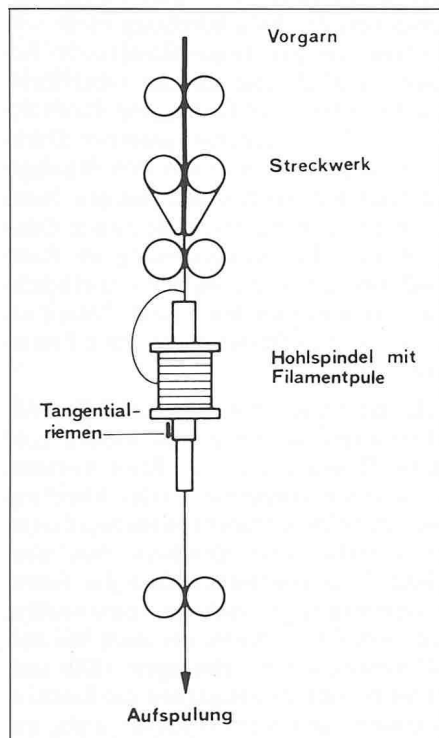
Bild 6. Umwindsprinzip: Coverspun
