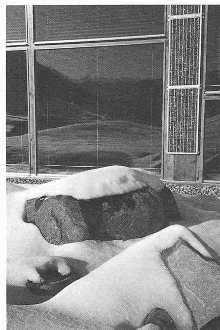
Bild 3. Detail des Fassadenkollektors mit den Sonnenzellen des Gleichstrom-Ventilators
