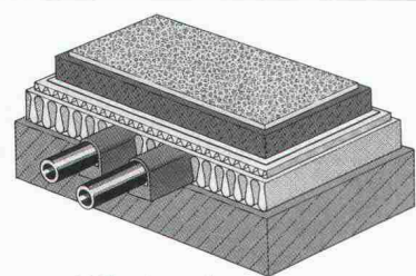
Fußbodenaufbau mit montierter Missel Kompakt-Dämmhülse
